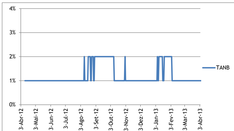
Simulação da TANB para o “Depósito Indexado Millennium Cabaz Step Up” com base em dados históricos
