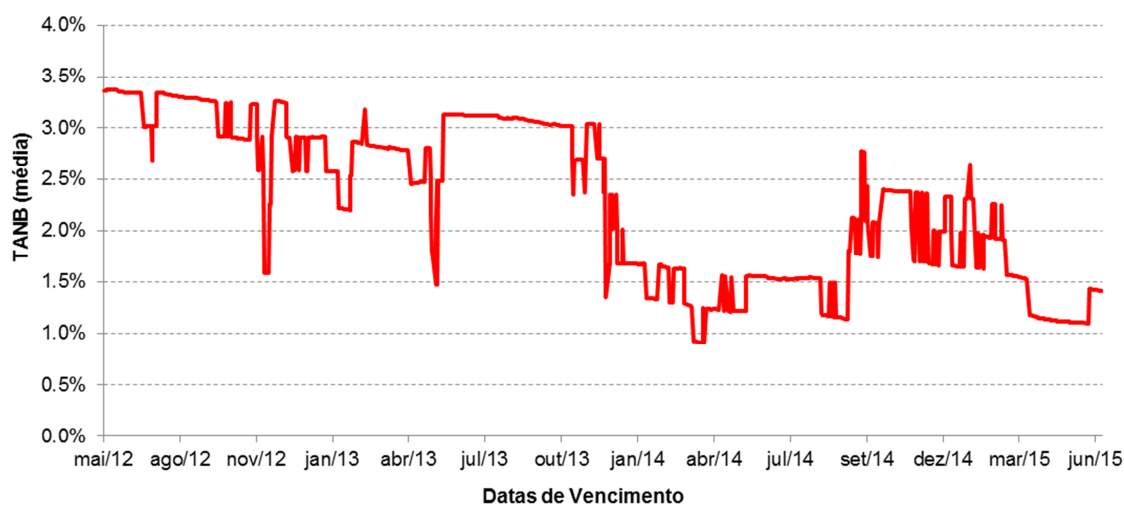
Depósito Indexado "Depósito Valor Acções EUA" Simulação da TANB (média) com base em dados históricos (Depósitos vencidos entre 18 de Maio de 2012 e 18 de Junho de 2015)
