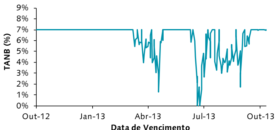
Simulação da TANB do depósito "Invest Super Brands (Ser. 13/1)" com base em dados históricos
