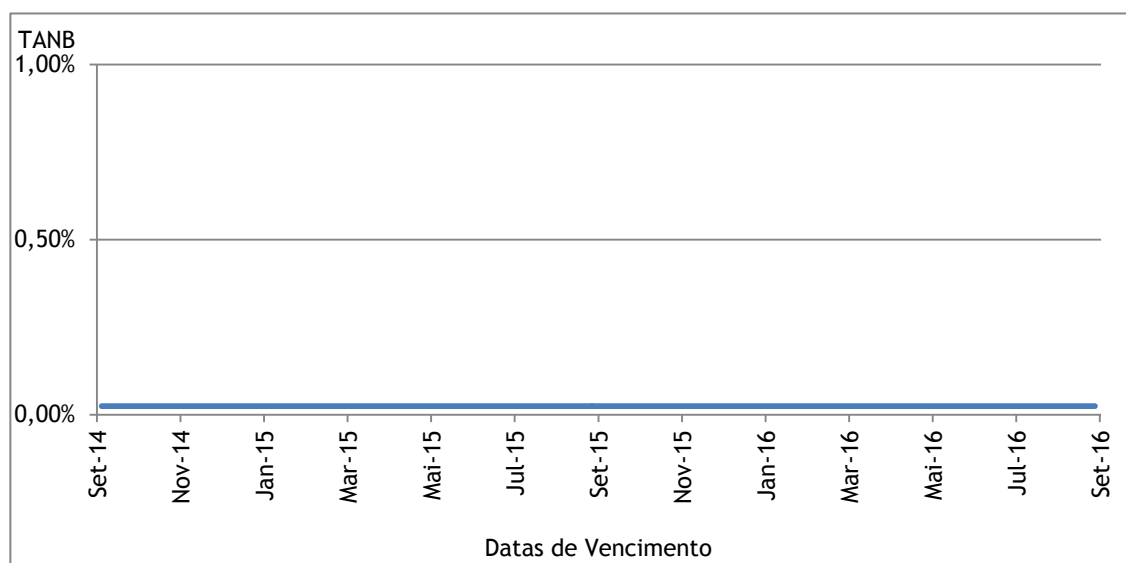
Simulação da TANB para o Depósito Indexado “Millennium Cabaz Universal outubro 2018” com base em dados históricos (depósitos vencidos entre os dias 1 de setembro de 2014 e 1 de setembro de 2016)
