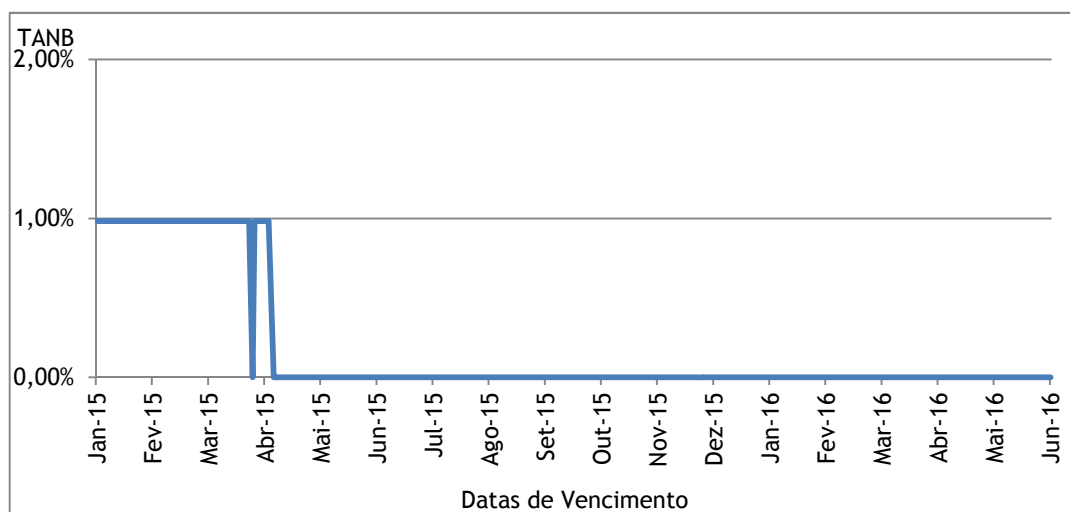
Simulação da TANB para o Depósito Indexado “Millennium Mix Cabaz Global fevereiro 2018” com base em dados históricos (depósitos vencidos entre os dias 2 de janeiro de 2015 e 29 de junho de 2016)
